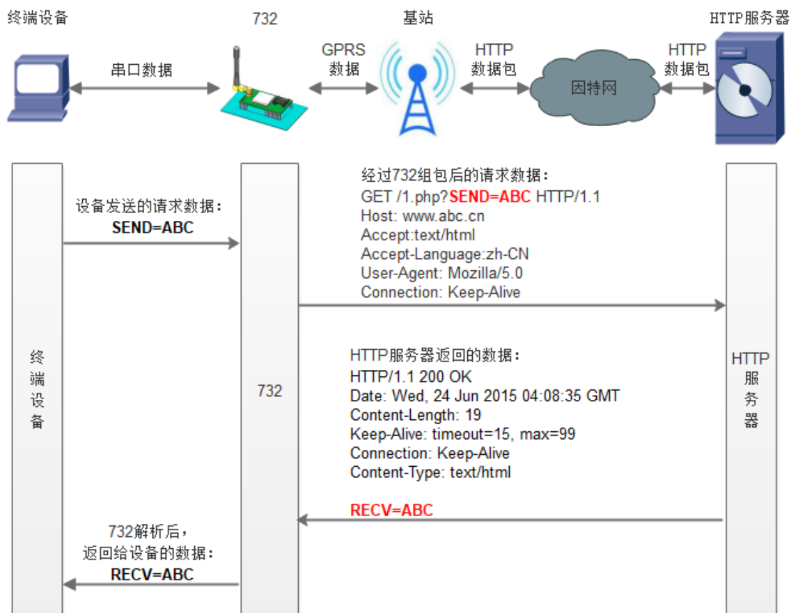
图 4 HTTPD 模式
