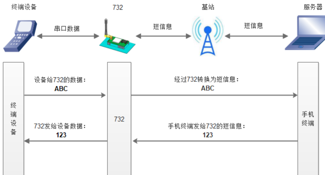
图 7 短信透传模式
