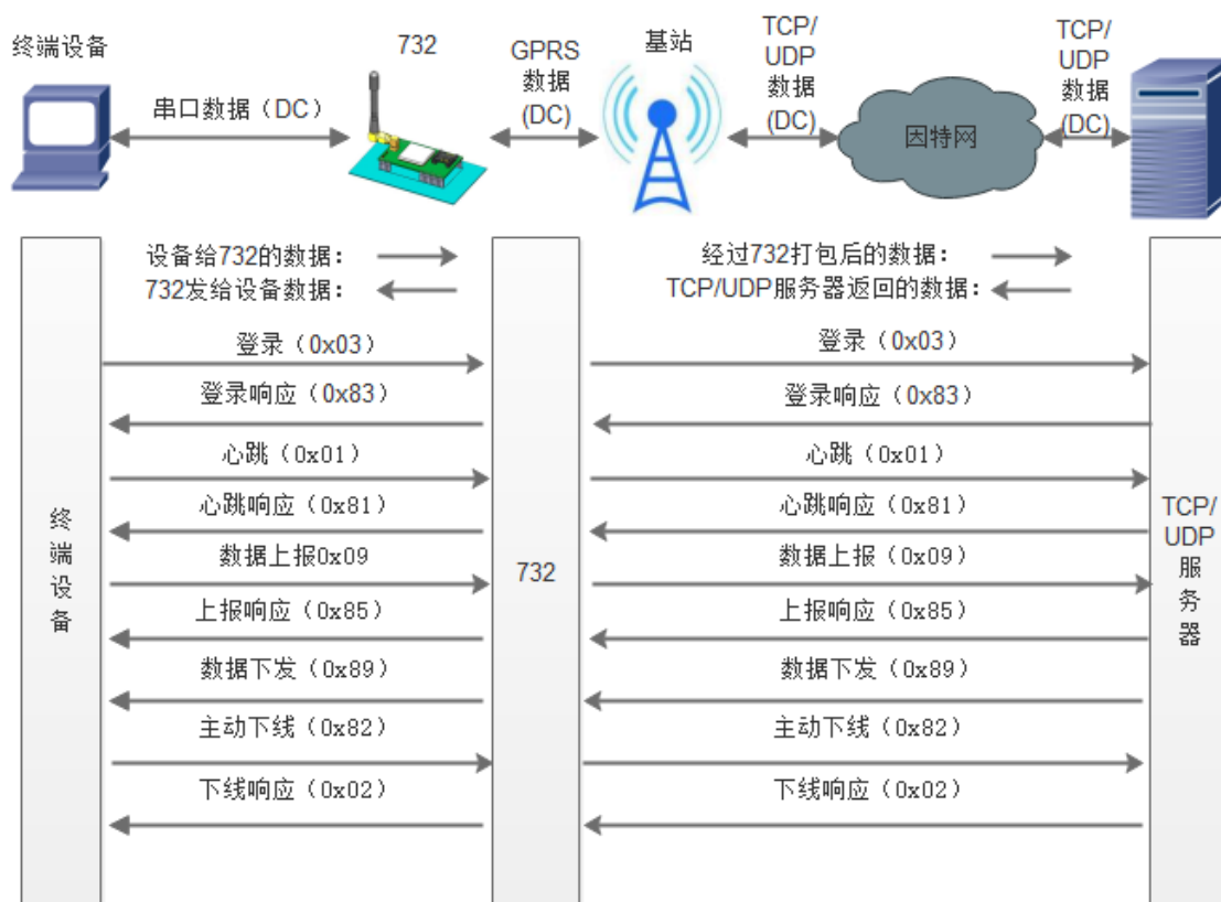
图 9 UDC 模式
