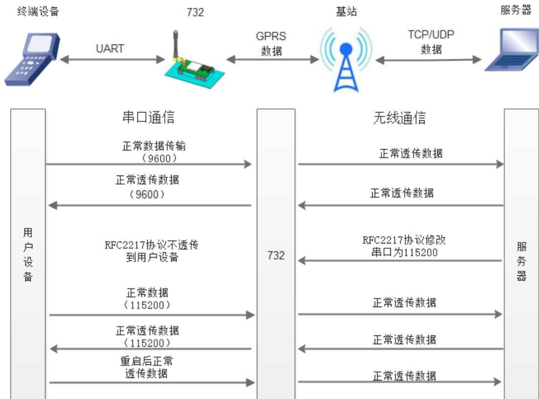
图 12 类 RFC2217 功能逻辑示意图
