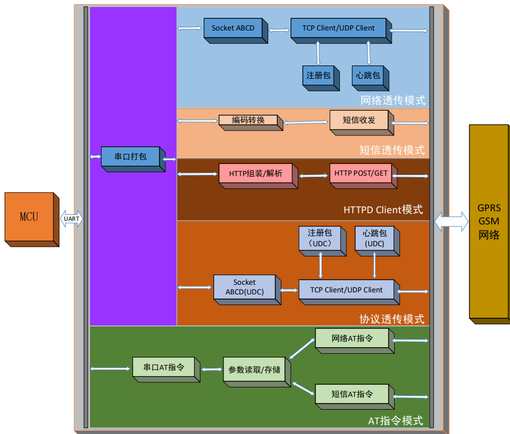
图 1 功能框图
