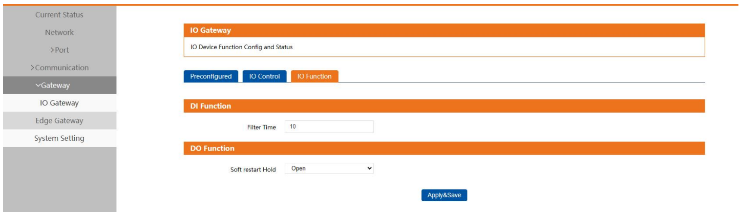
Fig. 22 IO function
